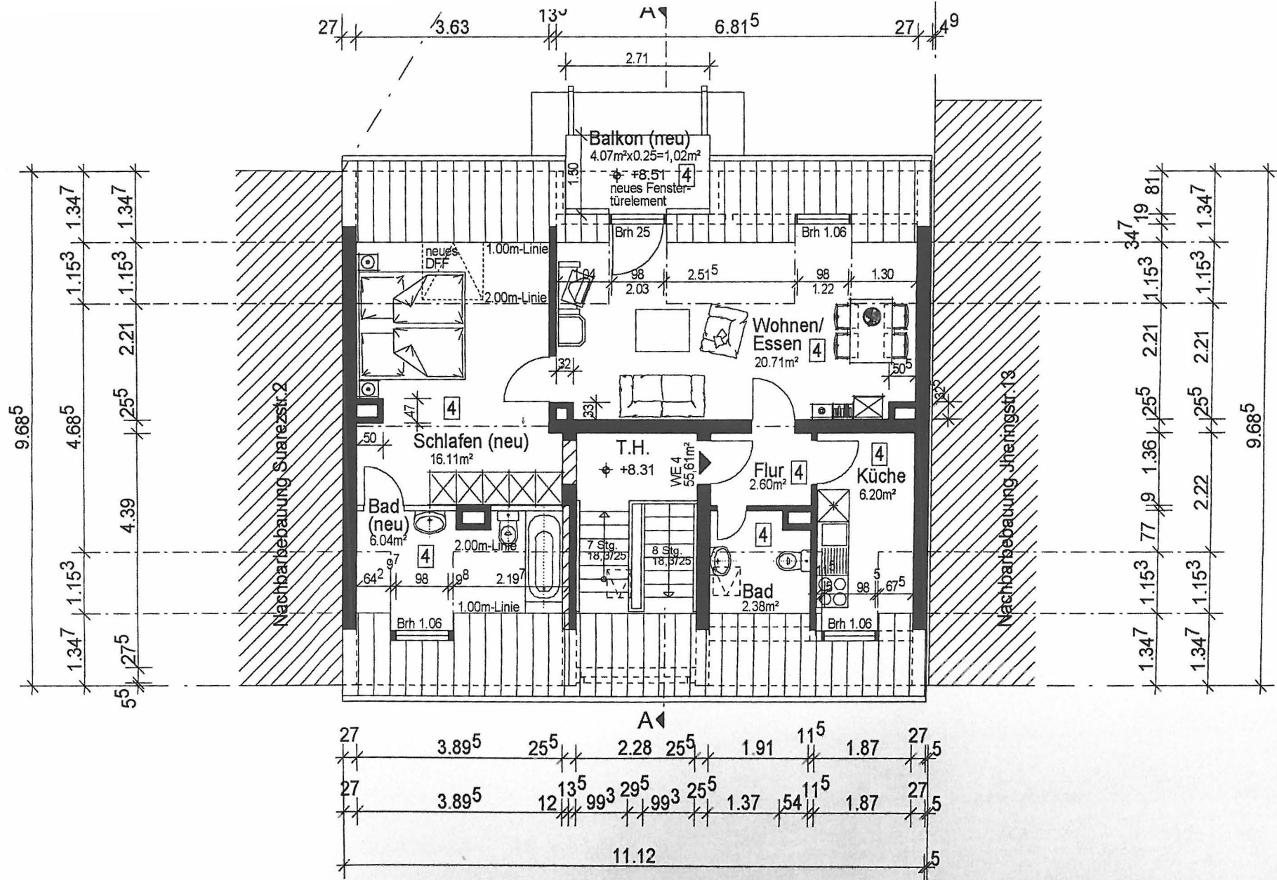
Dachgeschoß
